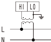
电压经互感器接入
