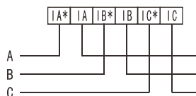
电流直接接入
