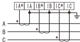
电流经互感器接入
