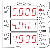
图1：分相电流 (A) 显示
