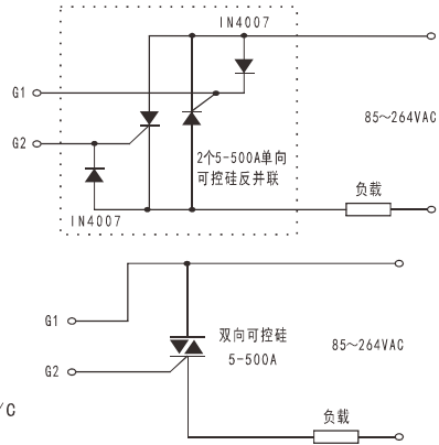
可控硅触发出线线图
