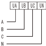
电压直接接入 (nEt=n3. 4)
