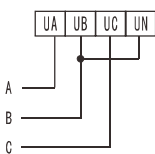
电压直接接入 (nEt=n3. 3)
