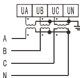
电压经互感器接入 (nEt=n3. 4)
