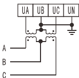
电压经互感器接入 (nEt=n3. 3)
